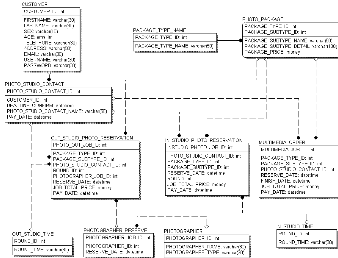
รูปที่ 7-2 ER Diagram ระบบ สตูดิโอถ่ายภาพ
